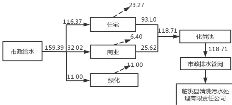
图 2-1 项目水平衡示意图 单位：m 3 /d
